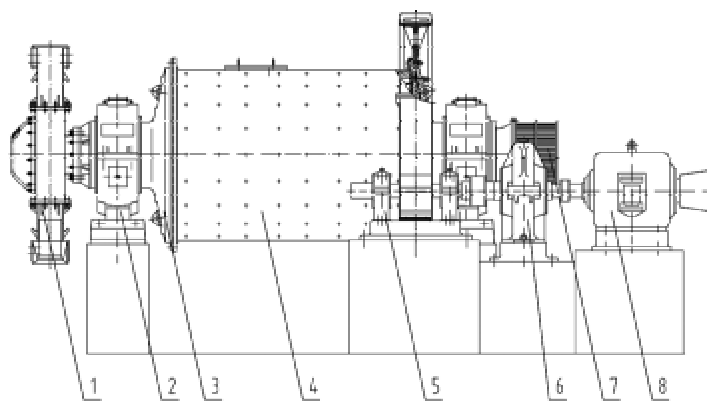
1. 联合给料部 2. 轴承部 3. 进料部 4. 筒体部 5. 传动部 6. 减速机 7. 出料部 8. 电动机
